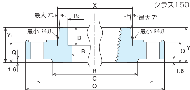
SW-RF形
