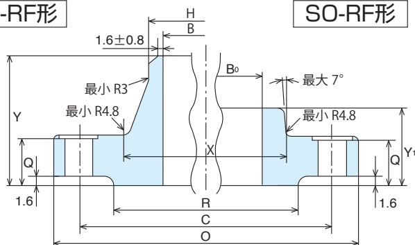
SW-RF形
